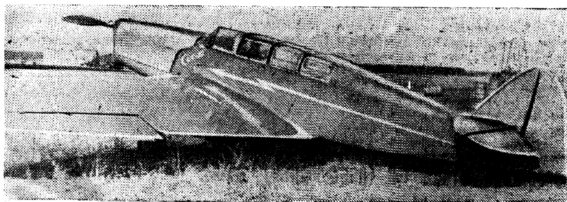
8 августа закончились испытания нового почтово-пассажирского скоростного самолета воронежского авиаконструктора А. С. Москалева „СМ-10“. Данные испытания показали исключительно высокие летные качества „СМ-10“. По своим летным техническим качествам „СМ-10“ идет значительно впереди лучших зарубежных образцов („Симун Кодрон“ и др.). Новый самолет, наряду с высокими летными качествами, весьма дешев и прост в производстве. На снимке: самолет „СМ-10“.
