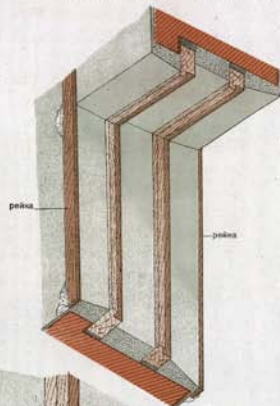
ОШТУКАТУРИВАНИЕ ОКОННОГО ПРОЕМА
