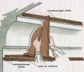
ОШТУКАТУРИВАНИЕ СТОЛБОВ ПО РЕЙКАМ
