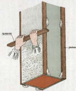
ОШТУКАТУРИВАНИЕ СТОЛБОВ ПО РЕЙКАМ
