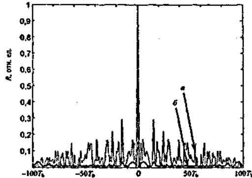
Рис. 1. Функции автокорреляции R(y) = \int E^*(x)E(x+y)dx сигнала со случайной бифазовой модуляцией (а) и сигнала Фрэнка (б), состоящих из N = 100 элементарных импульсов.
