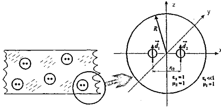
Рис. 4. Сферическая частица радиуса R , содержащая два атома с дипольными моментами \vec{d}_1 и \vec{d}_2 , помещенная в метаматериал с диэлектрической проницаемостью \epsilon_1 , |\epsilon_1| \ll 1 .
