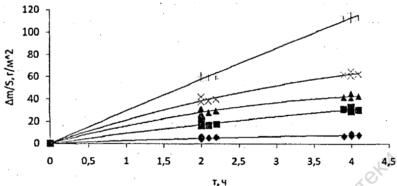
Рисунок 4 – Влияние времени термообработки при температуре 800°C на интенсивность окисления покрытий, содержащих Al и Ni: * – M1, ▲ – AD1, ◆ – AD1/HP2, × – (AD1+HP2), ■ – AD1/(AD1+HP2); R^2=0,89-0,99
