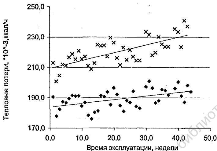
Рисунок 6 – Изменения тепловых потерь через воздушные фурмы в процессе эксплуатации: \blacklozenge – опытная фурма с АД1/Х20П80 покрытием, \times – серийная фурма с АД1 покрытием
