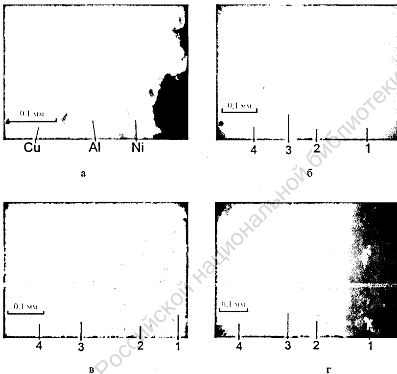
Рисунок 2 – Структура поверхностного слоя на медных образцах с АД1 / НП2 покрытием: а – после напыления; после термообработки: б – 700°С 6ч, в – 800°С 6ч, г – 900°С 6ч; участки, содержащие: 1 – Ni, 2 – Ni, Al, Cu; 3 – Al, Cu; 4 – Cu
