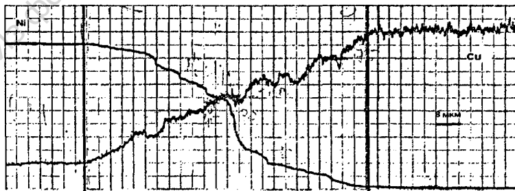
Рисунок 1 – Распределение Ni и Cu в диффузионном слое образца после термообработки
