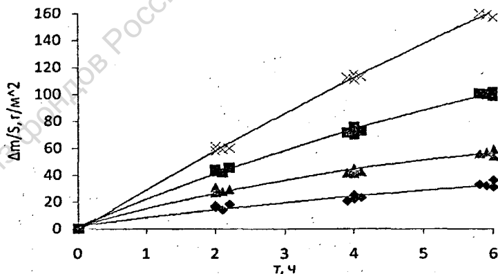
Рисунок 5 – Зависимость интенсивности окисления медных образцов от времени выдержки при температуре 800°C: × – М1, ■ – АХФ, ▲ – АД1, ◆ – АД1/АХФ; R^2=0,94-0,99
