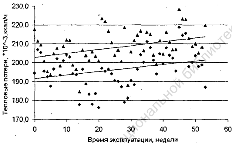
Рисунок 7 – Изменение тепловых потерь через воздушные фурмы в процессе эксплуатации: ♦ – опытная фурма с обмазкой, ▲ – серийная фурма с АД1 покрытием
