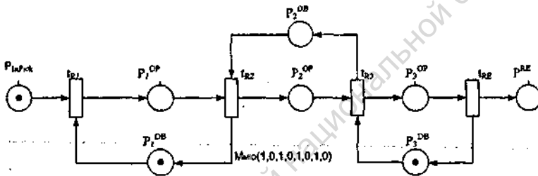
Рисунок 4. Модель последовательной реализации операции выборки в виде сети Петри.
