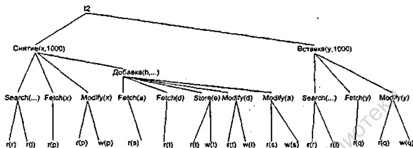
Рисунок 5. Пример слияния и декомпозиции двух транзакций по модели объекта транзакционного сервера
