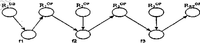
Рисунок 2. Модель в виде двухдольного графа основных типов операций, изменяющих состав или структуру БД
