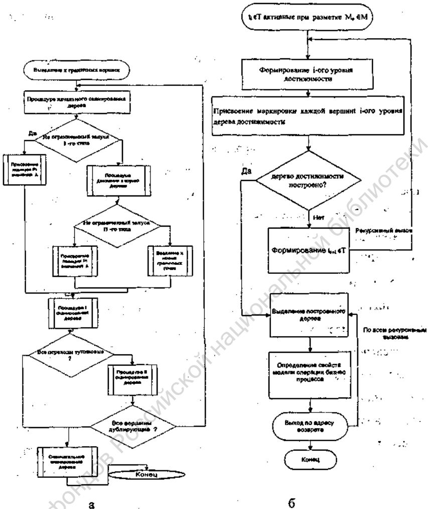
Рисунок 1.а. Итеративный алгоритм построения дерева достижимости,
