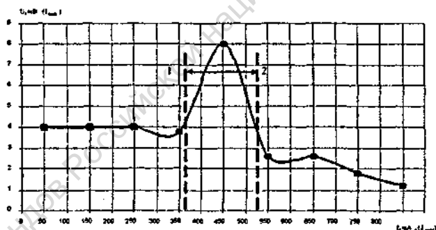
Рис. 2. Экспериментальная зависимость выходной интенсивности от входной: 1-2 – рабочий диапазон
