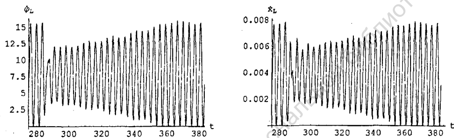
Рис. 7: Срыв установившегося автоколебательного режима
