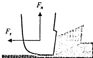
Рис. 1: Резец, вырезающий канавку постоянного сечения
