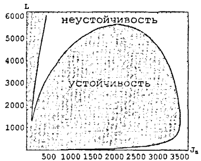
Рис. 5: Зоны устойчивости и неустойчивости в низкочастотной области
