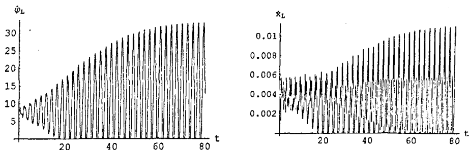
Рис. 6: Установление близкого к периодическому режима с этапами застоя долота
