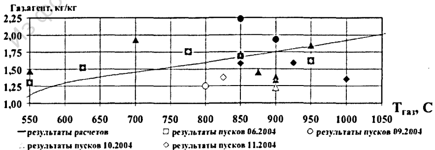
Рис.3. Сопоставление экспериментальных и расчетных параметров реактора
