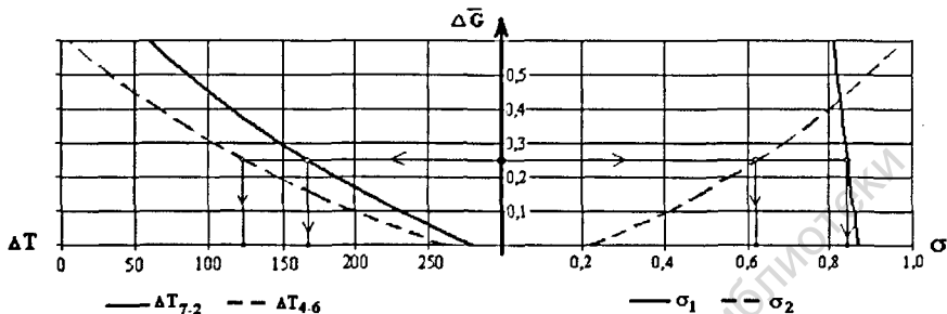
Рис. 10. Номограмма эффективности теплообменного аппарата по уравнениям (1)...(4) для осушенного газа ( T_5=1273 К, C_{p1}=1,133 кДж/(кг·К), G_1=0,86 кг/с)
