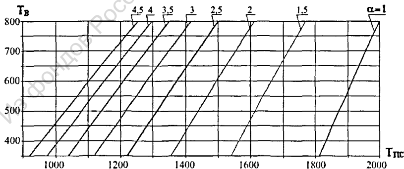
Рис. 5. Температура сгорания генераторного газа - продукта газификации ТБО, (газ осушен, температура генераторного газа на входе в камеру сгорания 300 К)
