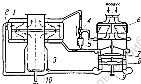
Рис. 11. Принципиальная схема энерготехнологической ГТУ: 1 - высокотемпературный двухъярусный воздухонагреватель, 2 - регулятор перепуска байпасного воздуха, 3 - основная камера сгорания, 4 - блок регулирования перепуска холодного воздуха, 5 - пусковая камера сгорания на пусковом топливе, 6 - двухкаскадный компрессор со встроенным воздухоохладителем, 7 - турбина привода компрессоров, 8 - силовая турбина, 9 - муфта привода электрогенератора, 10 - горелка
