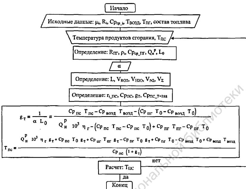
Рис 4. Блок-схема расчёта характеристик продуктов сгорания генераторного газа
