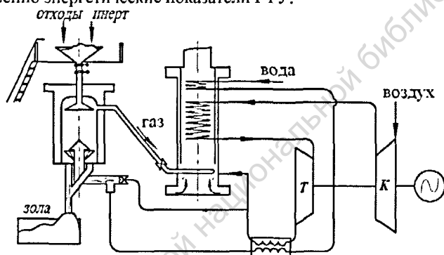
Рис. 7. Схема ГТУ на твердых горючих (разработка МГТУ им. Баумана)
