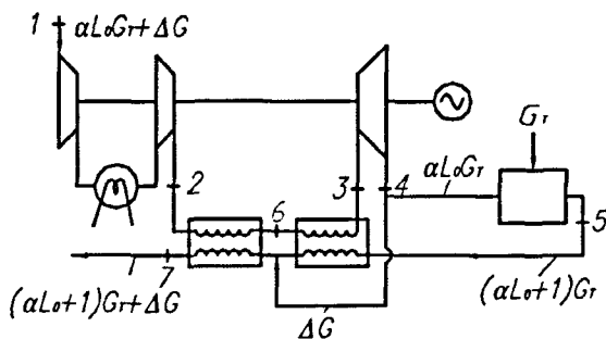
Рис. 8. Модифицированная схема ГТУ
