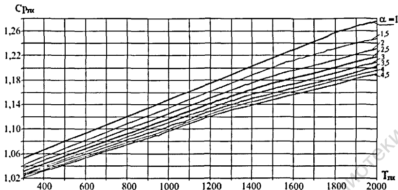
Рис. 6. Средняя теплоемкость продуктов сгорания осушенного генераторного газа-продукта газификации ТБО
