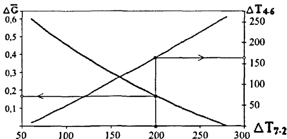
Рис. 9. Номограмма для расчета относительной массы перепуска ( T_3=1273 К, L_0=1,28 , \alpha=3,89 , Cp_l=1,133 кДж/(кг·К), G_T=0,86 кг/с)
