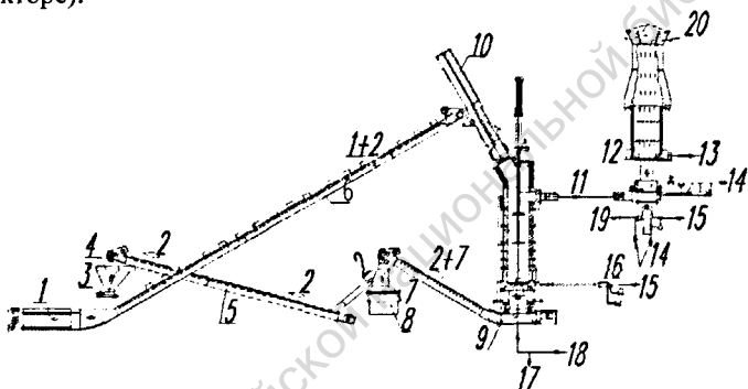
Рис. 1. Технологическая схема комплекса с реактором-газификатором на площадке ФГУП ММП «Салют»; 1 – сырье, 2 – инерт, 3 – конвейер подачи инерта с весами, 4 – воронка сбора инерта, 5 – конвейер подачи инерта в воронку, 6 – конвейер подачи сырья, 7 – зола, 8 – контейнер сбора золы, 9 – конвейер отвода золы с инертном от реактора, 10 – питающий механизм, 11 – продукт-газ, 12 – продукты сгорания продукт-газа, 13 – воздух на охлаждение продуктов сгорания продукт-газа, 14 – воздух на горение, 15 – легкое нефтяное топливо, 16 – блок розжига, 17 – пар, 18 – воздух, 19 – дежурное топливо, 20 – дымовая труба
