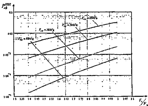
Рис. 5 Характеристики вероятности ложной фиксации ИПД
