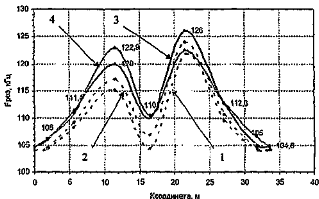
Рис. 2 Изменение резонансной частоты шлейфа в форме "восьмерка" при воздействии шунтами и реальным вагоном
