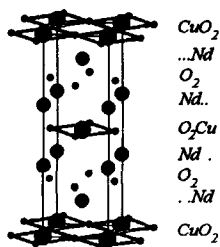
Рис. 7. Схема кристаллической структуры Nd_2CuO_4 .
