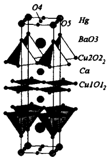
Рис. 4. Схема кристаллической структуры Hg-1223. Слои \text{Cu}_1\text{O}_1 и \text{HgO}_8 – плоские. Слои \text{Cu}_2\text{O}_2 – слегка гофрированы. В слое \text{HgO}_8 анионы могут частично занимать позиции O4 и O5 (позицию O5 – при частичном замещении Hg на Cu).
