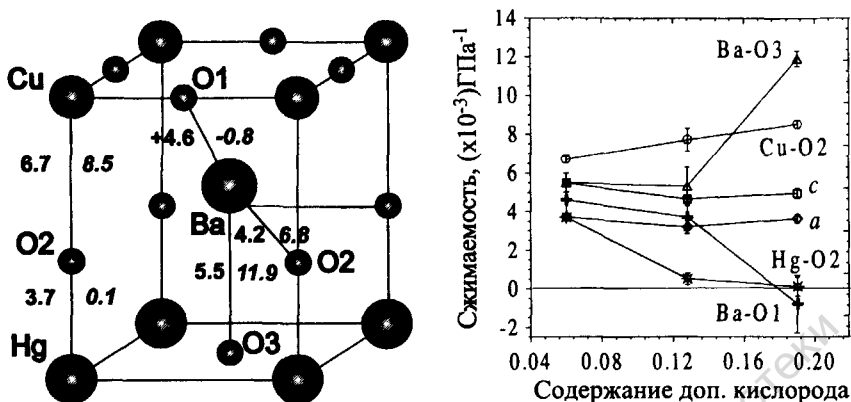
Рис. 3. На левом рисунке - схематическое изображение половины элементарной ячейки кристаллической структуры Hg-1201. Величины сжимаемостей некоторых длин связей в кристалле приведены слева для недодопированного, а справа - для передопированного образцов. На правом рисунке - зависимости сжимаемостей от содержания сверхстехиометрического кислорода.
