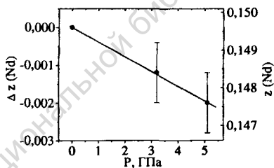
Рис. 9. Зависимость позиционного параметра z атома неодима (правая ось ординат) от давления. Прямая линия – линейная аппроксимация зависимости. На левой оси ординат отложена величина абсолютного изменения координаты.
