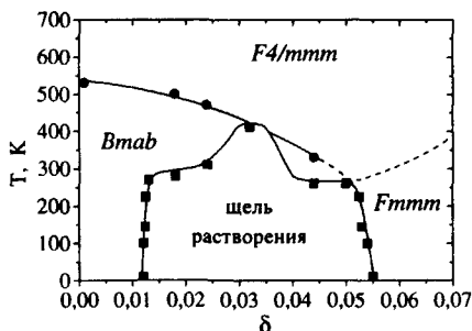
Рис. 10. Типичная фазовая диаграмма La_2CuO_{4+\delta} (рисунок скопирован из работы [11]). Кружочки и квадраты указывают температуры ОТ-перехода (из орторомбической в тетрагональную фазу) и фазового разделения, соответственно (по нейтрон-дифракционным данным). Штриховые линии отвечают предположительным (непроверенным еще) фазовым переходам. “Щель растворения” – область, в которой наблюдается разделение на богатую и бедную кислородом фазы
