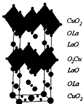
Рис. 11 Схема кристаллической структуры La_2CuO_4 .
